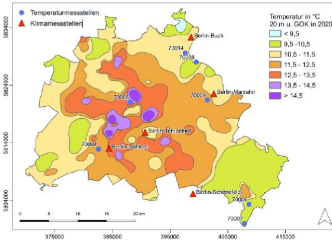
Grundwassertemperatur Berlin 2020
